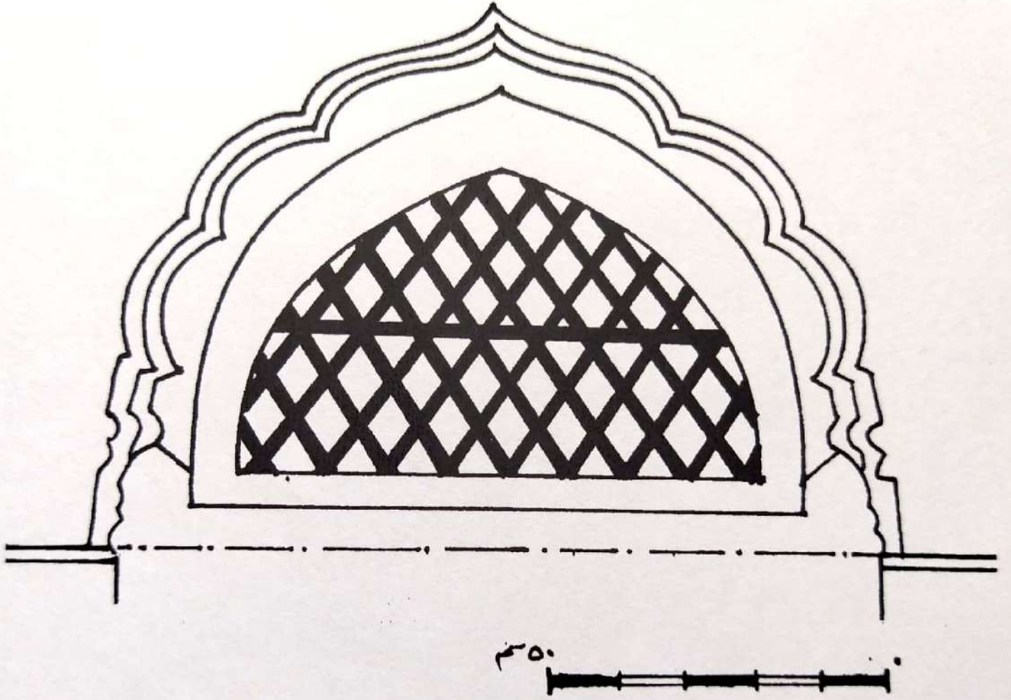
شكل ٢١ - شمسية من الطين المحروق المطلبي بالنورة تعلو الباب الشمالي الذي يتوسط البلاطة الوسطى بالطرف الغربي من رواق القبلة الحديث . يحيط بها أطر مفصصة
