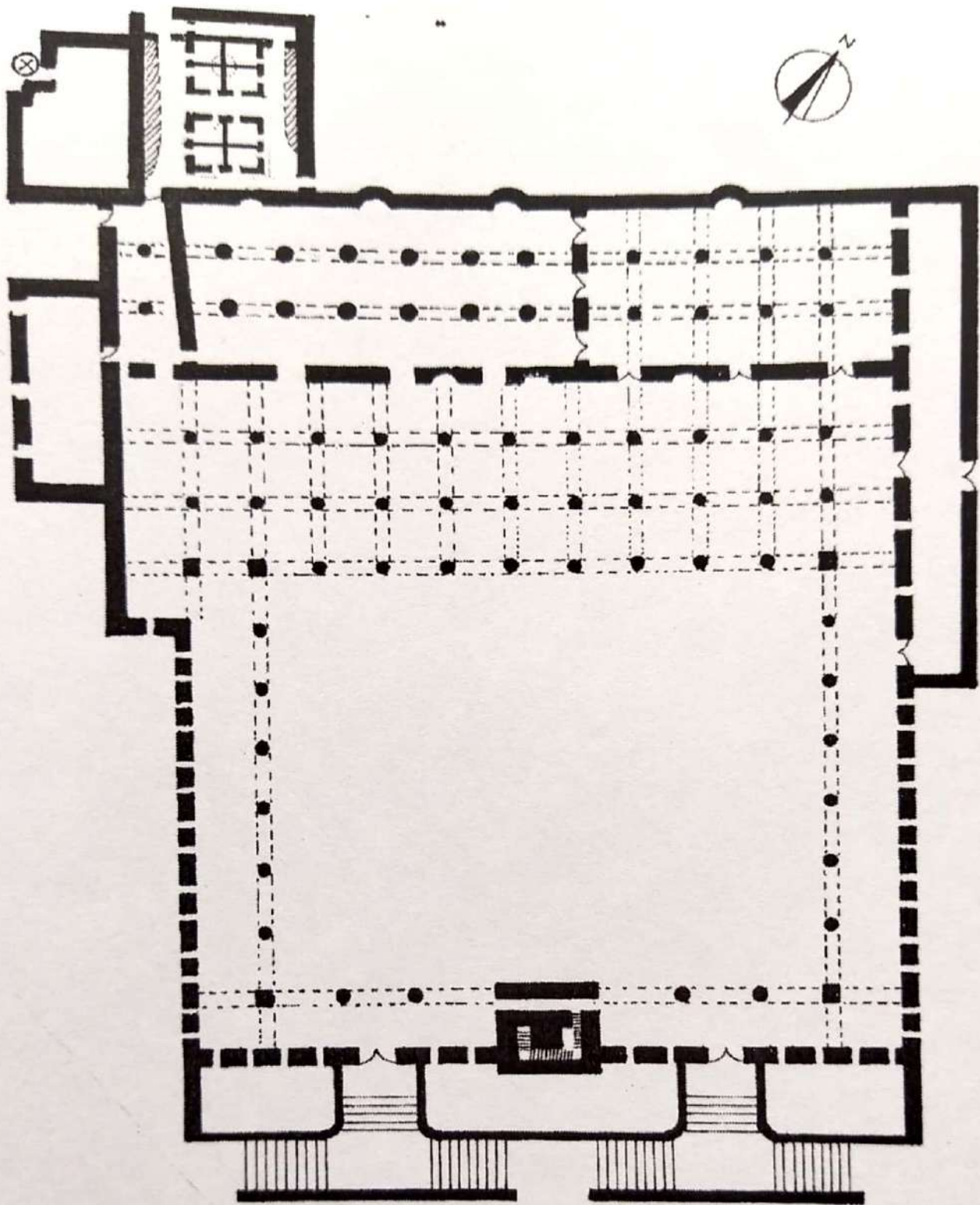
مسقط أفقي لمسجد الباحث - الباحت ١٩٩٤م
