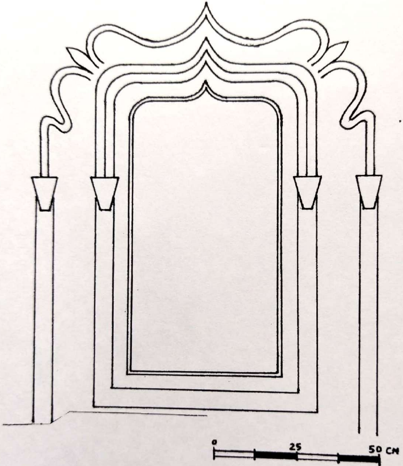
( شكل ٥ ) إحدى مشاكي قاعدة المئذنة
